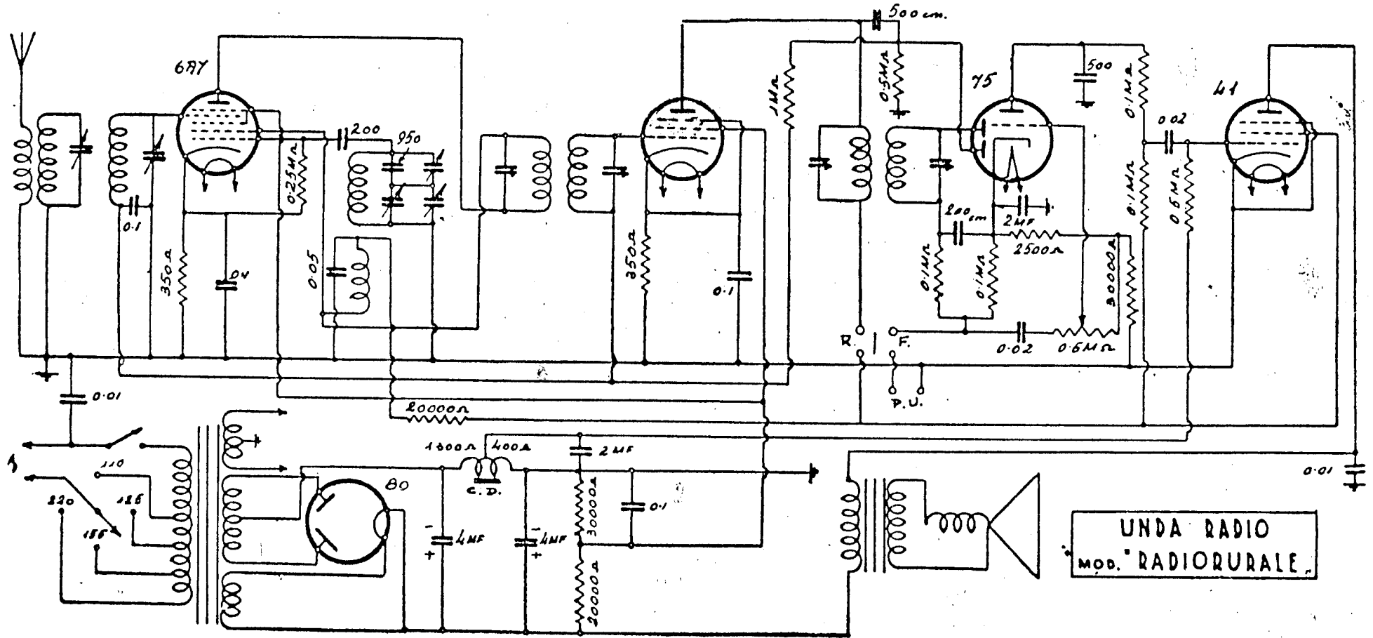
80. — Onde medie. - M. F. 175 kc. - C. A. V. - 6A7 oscill.-modul.; 78 amplif. m. f.; 75 demodul.-c.a.v.; 41 amplif. finale di potenza. - Scala parlante. - Presa per secondo altoparlante. - Potenza d'uscita: 2,5 watt.
